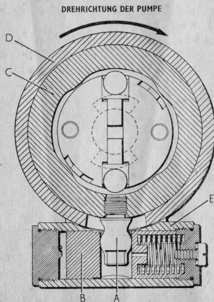
Abb. 5 Automatischer Einspritzmoment-Versteller
