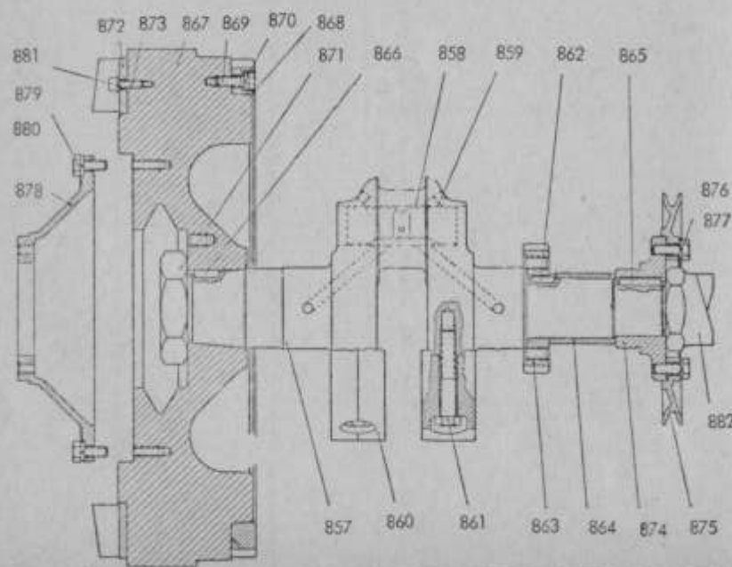
Kurbelwelle
