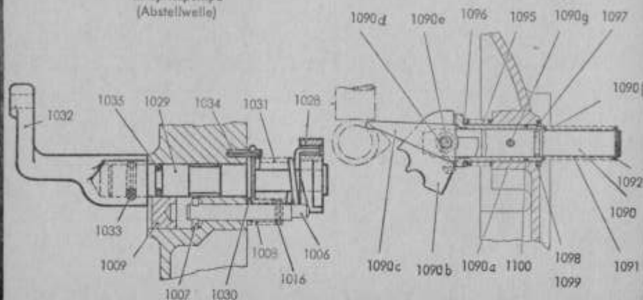
Einspritzpumpe (Abstellwelle)
