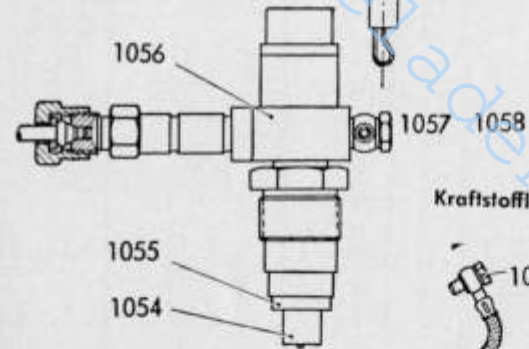
Einspritzventil
