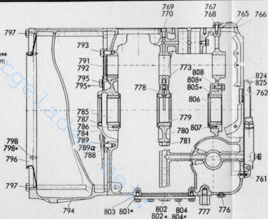
Kurbelgehäuse (Spiralgehäuse, Ansicht von hinten)
