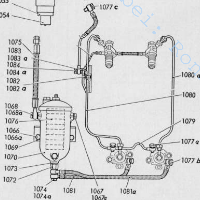
Kraftstoffleitungen bei angebaufem Filter
