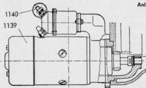
Anlasser
