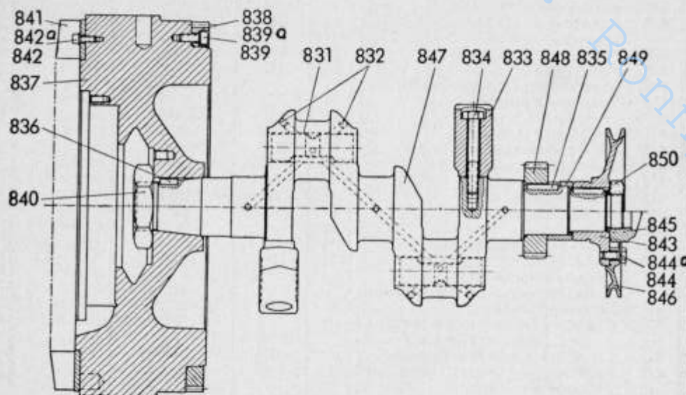
Kurbelwelle
