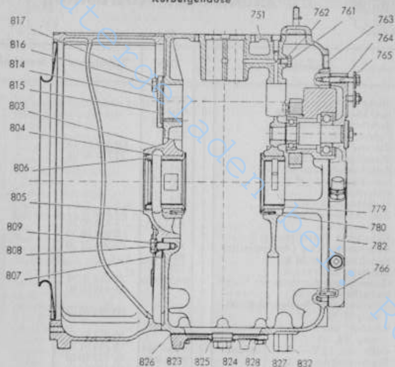
Kurbelgehäuse
