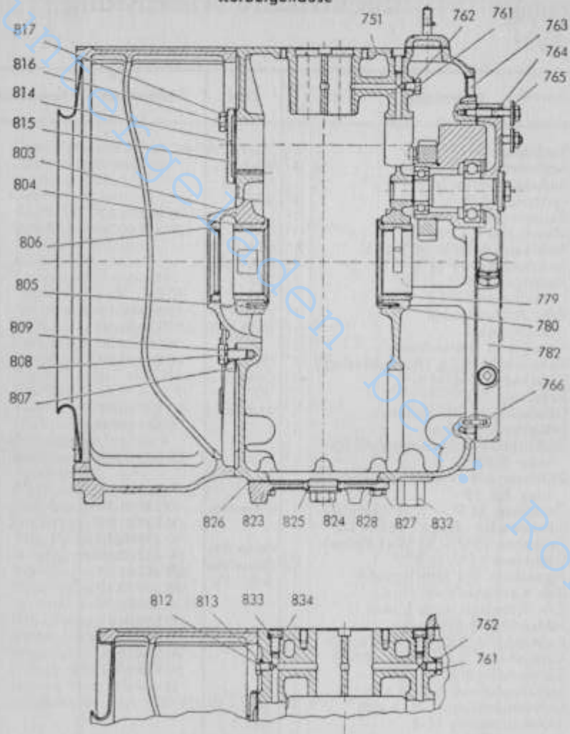
Kurbelgehäuse
