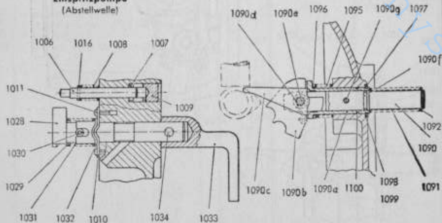
Einspritzpumpe (Abstellwelle)
